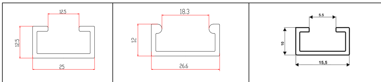
Supporto di fissaggio Tipo SAC25 Profilo per bordi tipo B1N - B2- B2N B1NC-AG - B2C-AG
