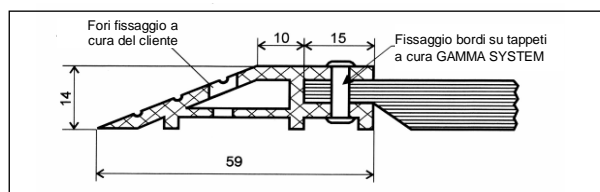
Profilo a scivolo tipo A
